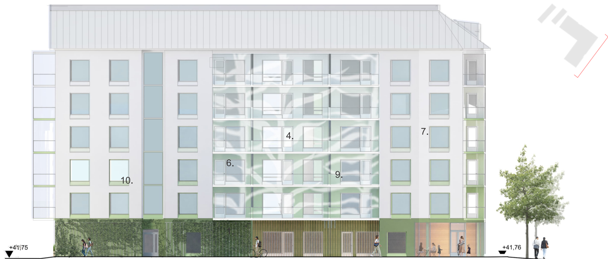
Julkisivu kaakkoon 1:200
